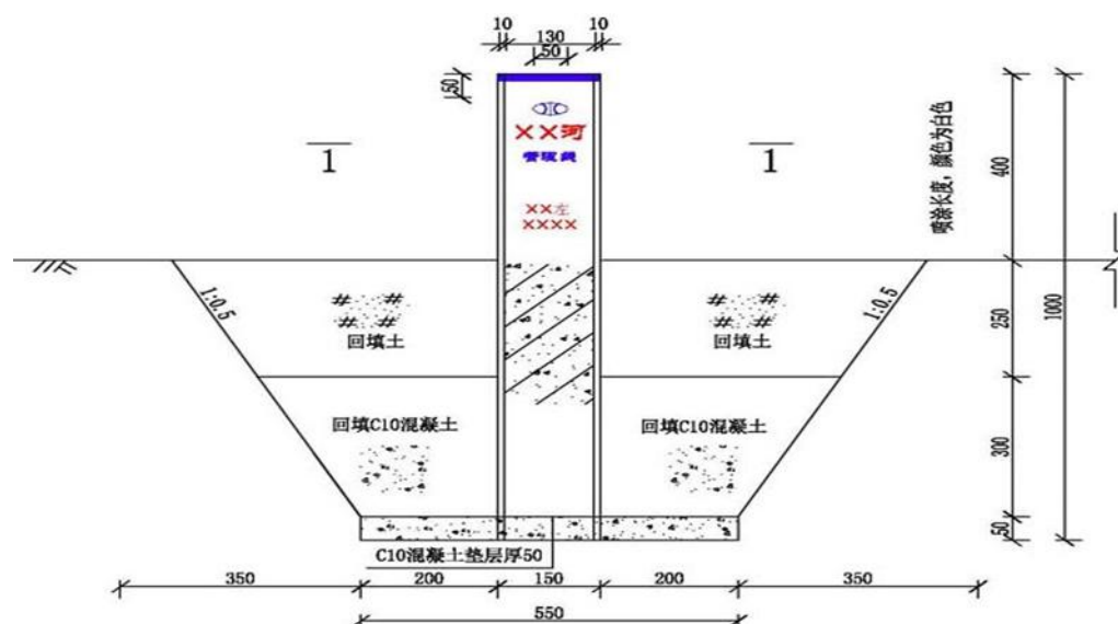
界桩结构图
