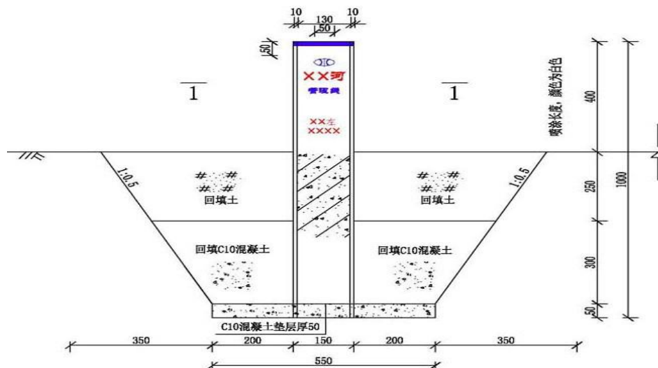
图4.7-1 界桩结构图
