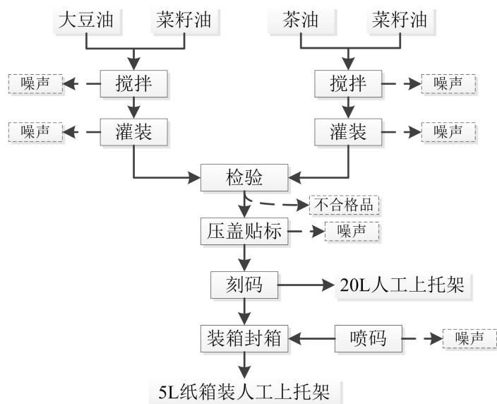
图 2.2-4 调和油灌装线工艺流程及产污节点图
