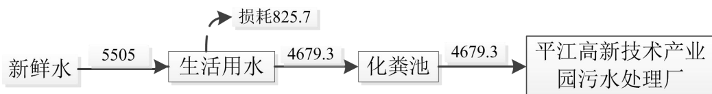
图 2.1-1 项目水平衡图（单位：m 3 /a）
