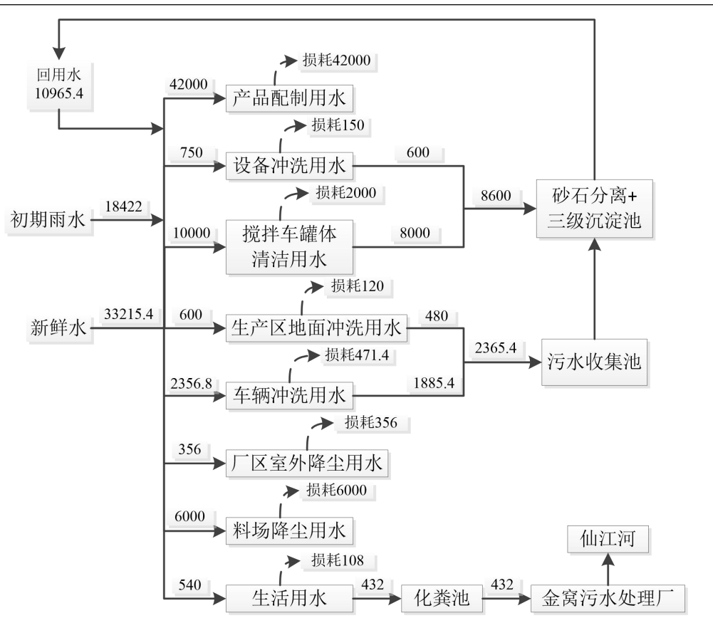
图 2.6-1 项目水平衡图 (单位: m³/a)
