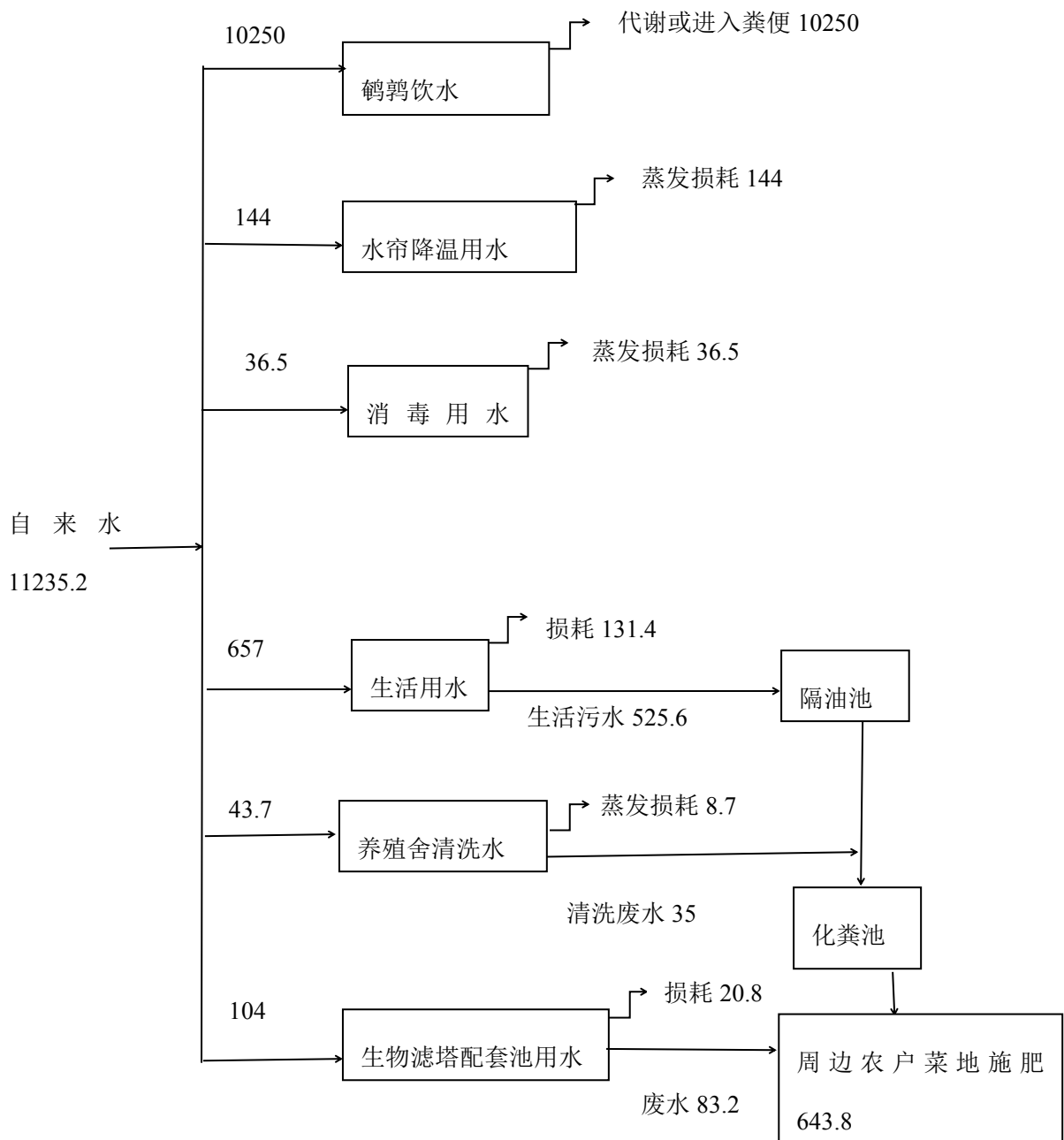
图 3.1-1 项目水平衡图 (单位: m³/a)
