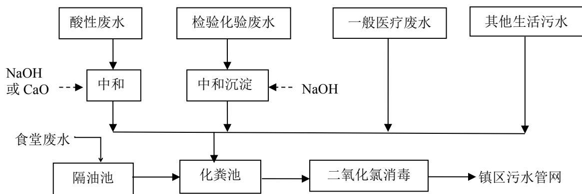
图 4-1 本项目污水处理工艺流程图
