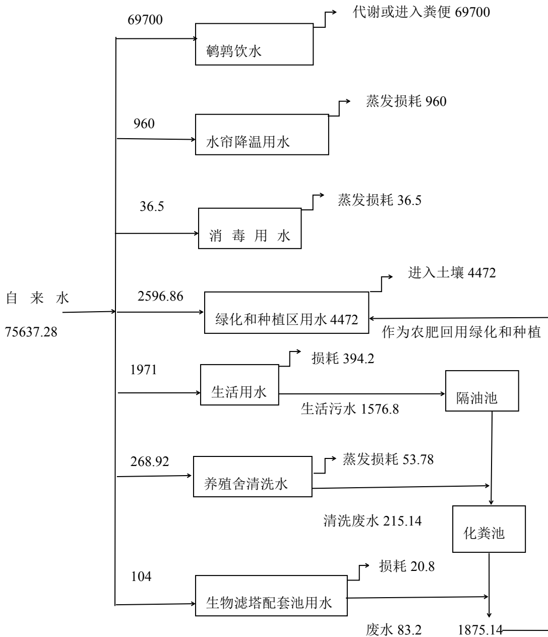
图 3.1-1 项目水平衡图 (单位: m³/a)
